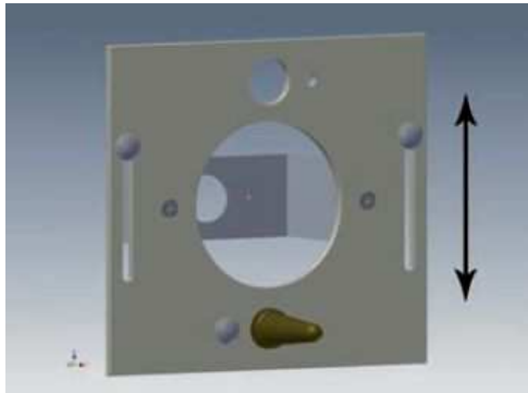
Предна плоскост с биберон, монтирана на височина за малки агнета.
